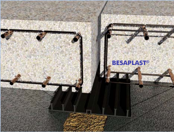
Anschweißbänder / waterstops for welding with sheets
