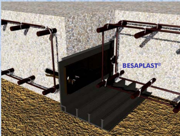
Klemmfugebänder / clamped waterstops
